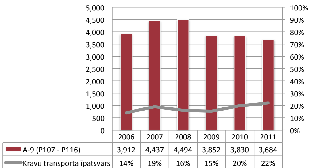
36. attēls. Satiksmes intensitātes dinamika A-9 (P109 – P116) Skrudas novadā
