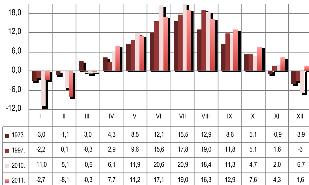
2. attēls. Vidējā mēneša gaisa temperatūra Skrudas novadā
