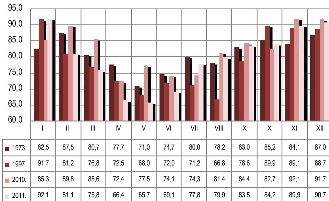
5. attēls. Vidējais mēneša relatīvais gaisa mitrums Skrudas novadā 1
