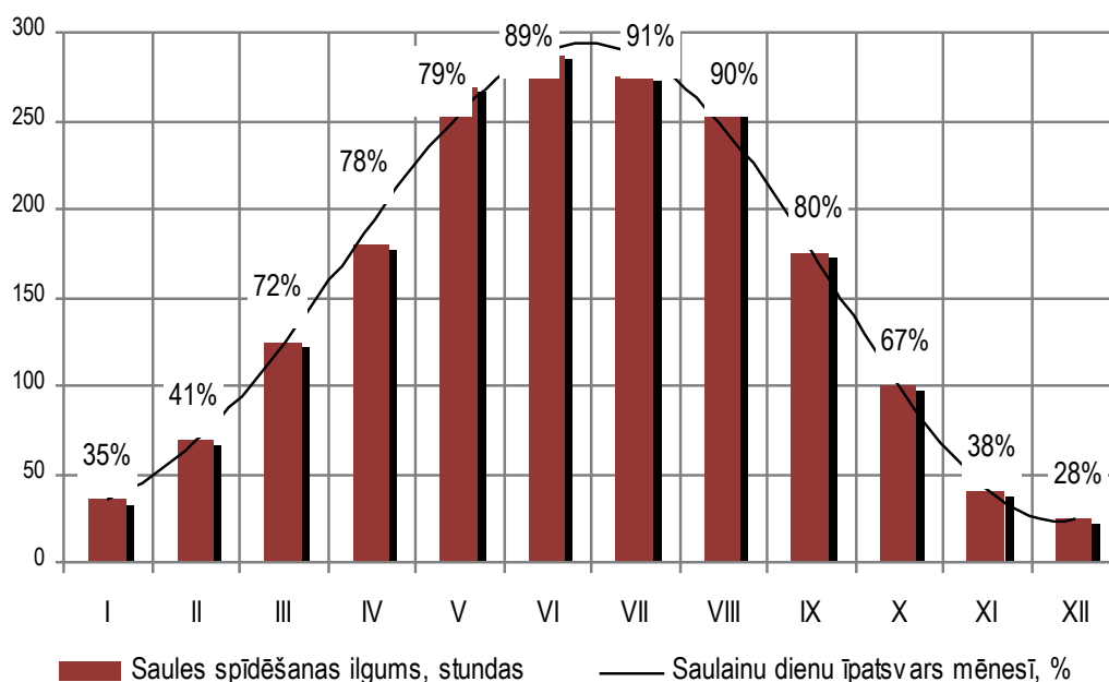
4. attēls. Saules spīdēšanas ilgums un saulaino dienu īpatsvars mēnesī Skrudas novadā (ilggadīgie dati)
