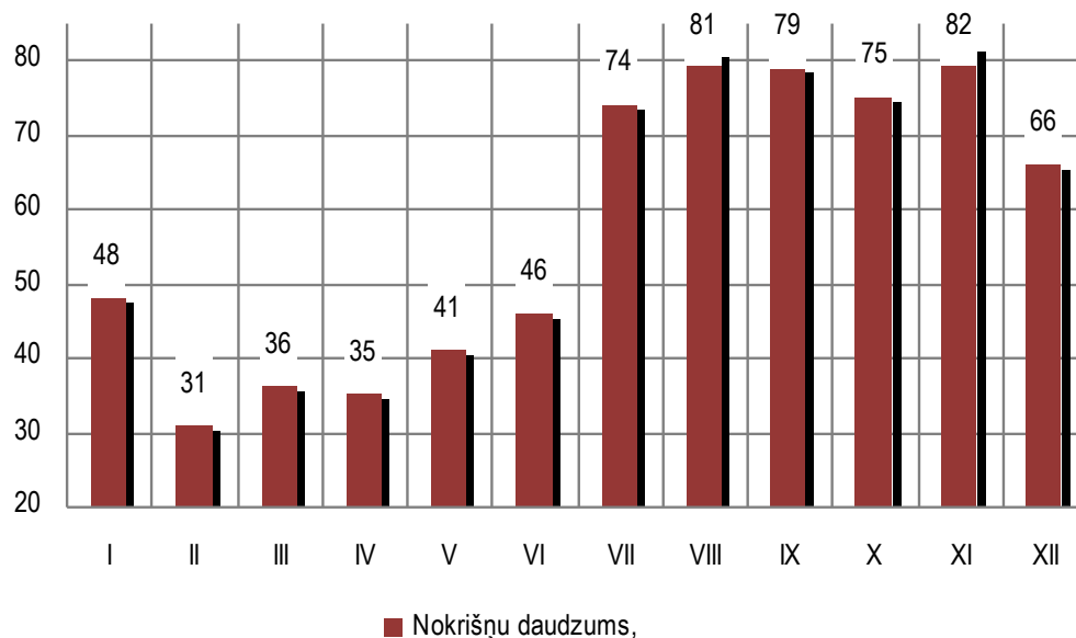
3. attēls. Ilggadīgais vidējais mēneša nokrišņu daudzums (mm) Skrudas novadā
